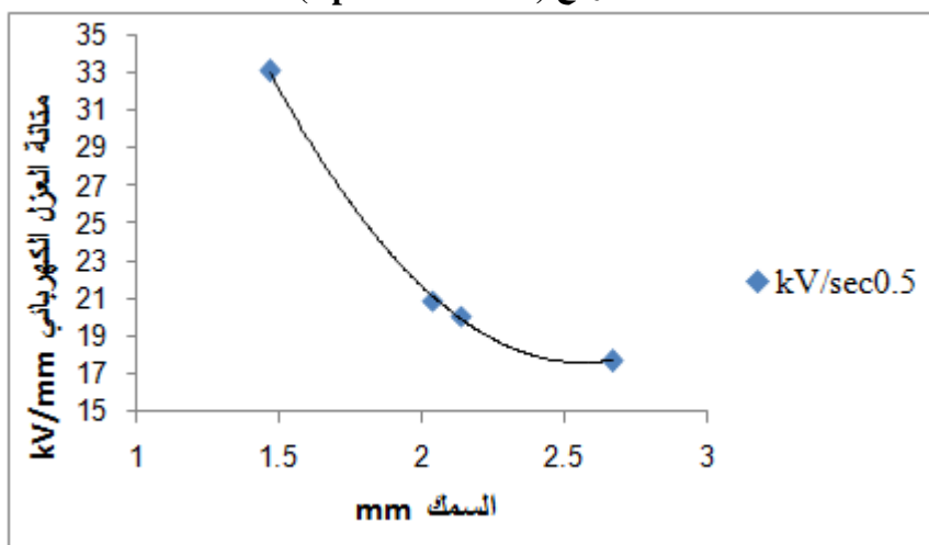
شكل (5) تغير السُمك مع متانة العزل الكهربائي للنموذج (Ep Pure)
