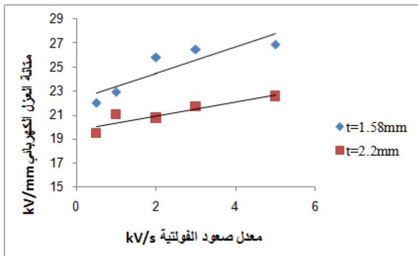
شكل (4) تغير متانة العزل الكهربائي مع معدل صعود الفولتية للنموذج (Ep + 15% SiO 2 )
