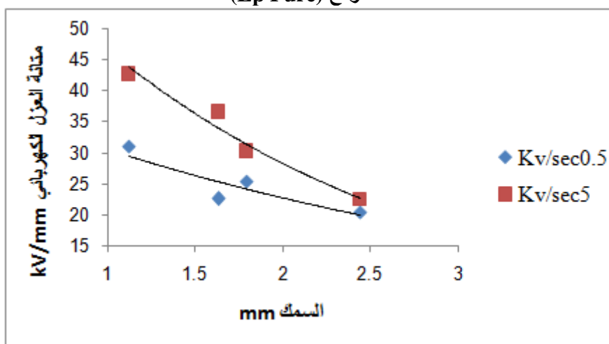
شكل (6) تغير السُمك مع متانة العزل الكهربائي للنموذج (Ep + 3.75% SiO 2 )
